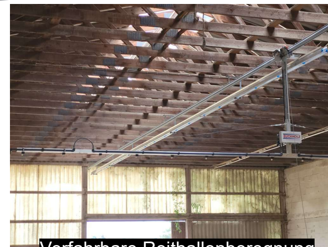
Verfahrbare Reithallenberegung
